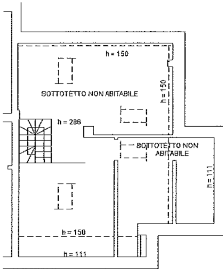
PIANO SOTTOTETTO
